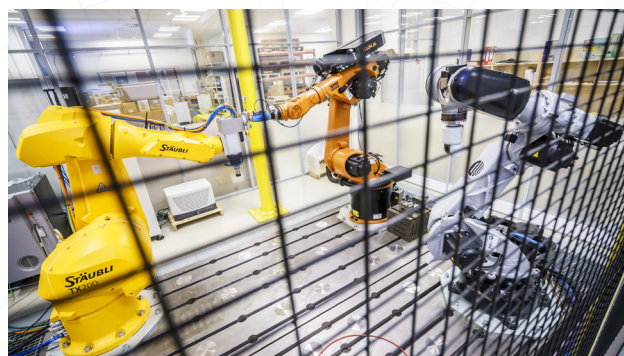
Pracoviště robotického obrábění
